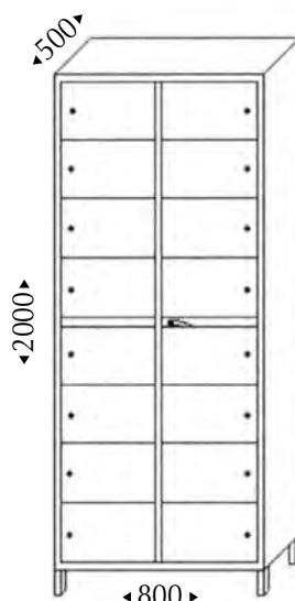
DH2 X 08 D (Toit droit)
