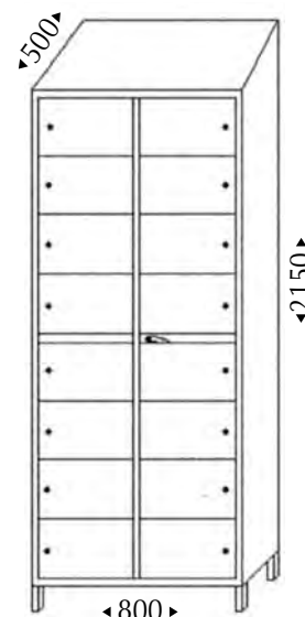
DH2 X 08 I (Toit incliné)
