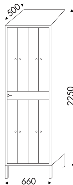
DV 82 I (Toit incliné)
