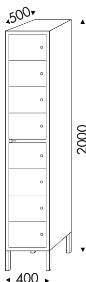
DH 08 D (Toit droit)
