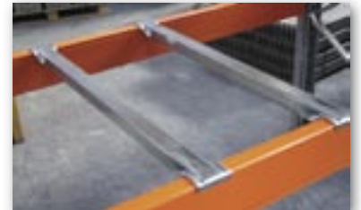
Traverse de stockage emboutie Ne convient pas pour les platelages aggro.
